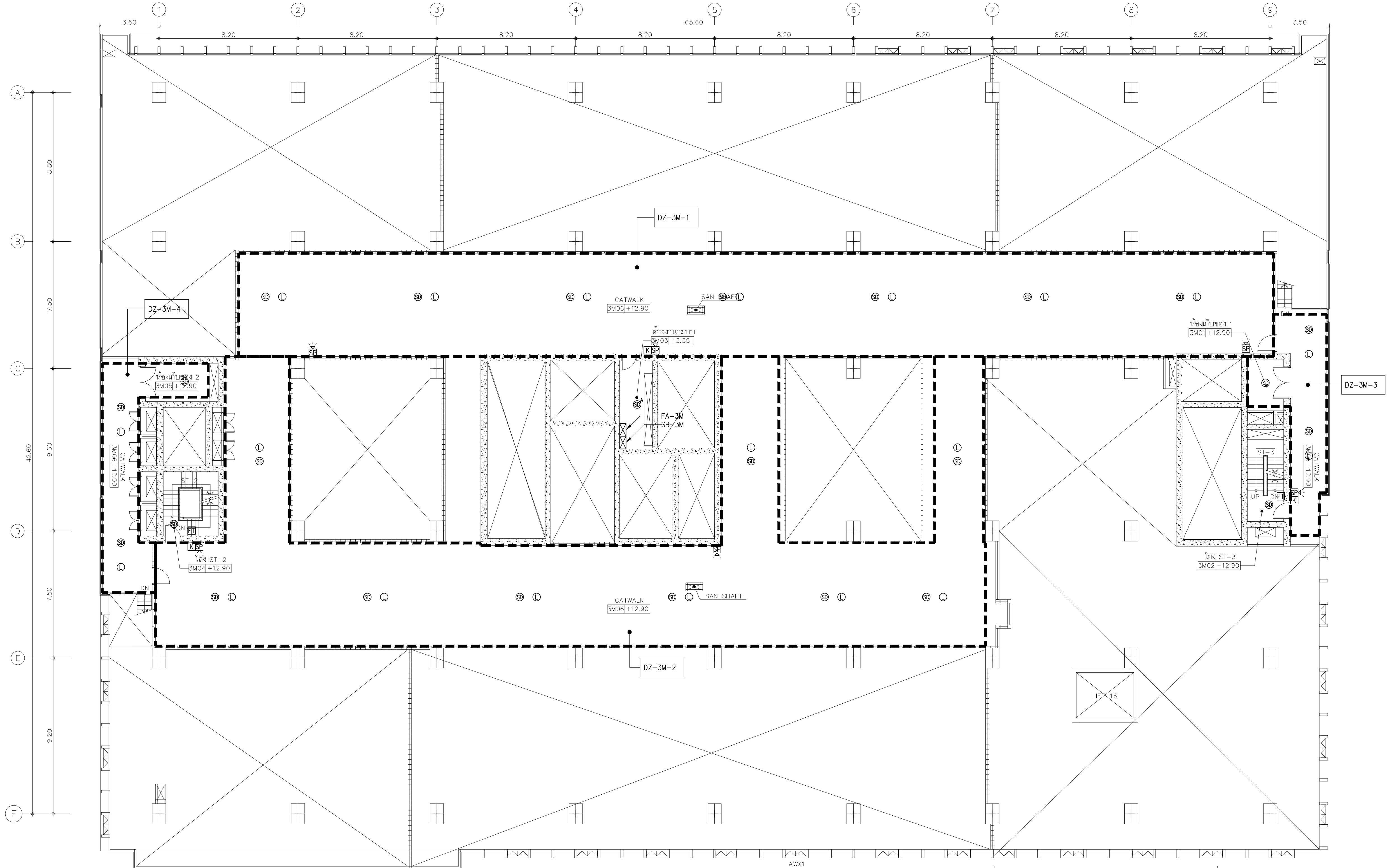
01 แปลนระบบแจ้งเหตุเพลิงไหม้และเสียงประกาศชั้นลอย 3M A1@ 1:125 A3@ 1:250
