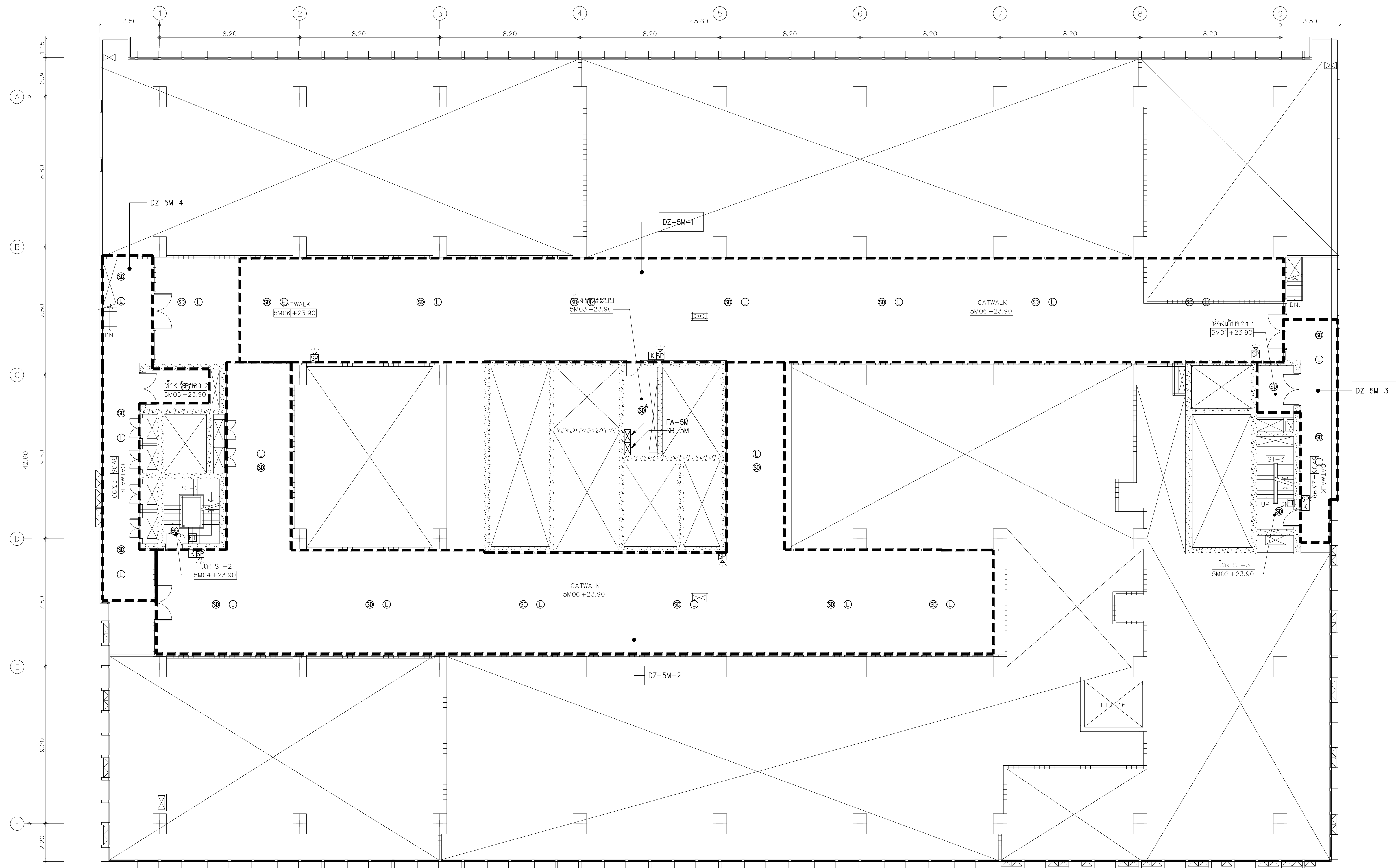
01 แปลนระบบแจ้งเหตุเพลิงไหม้และเสียงประกาศชั้นลอย 5M A1@ 1:125 A3@ 1:250
