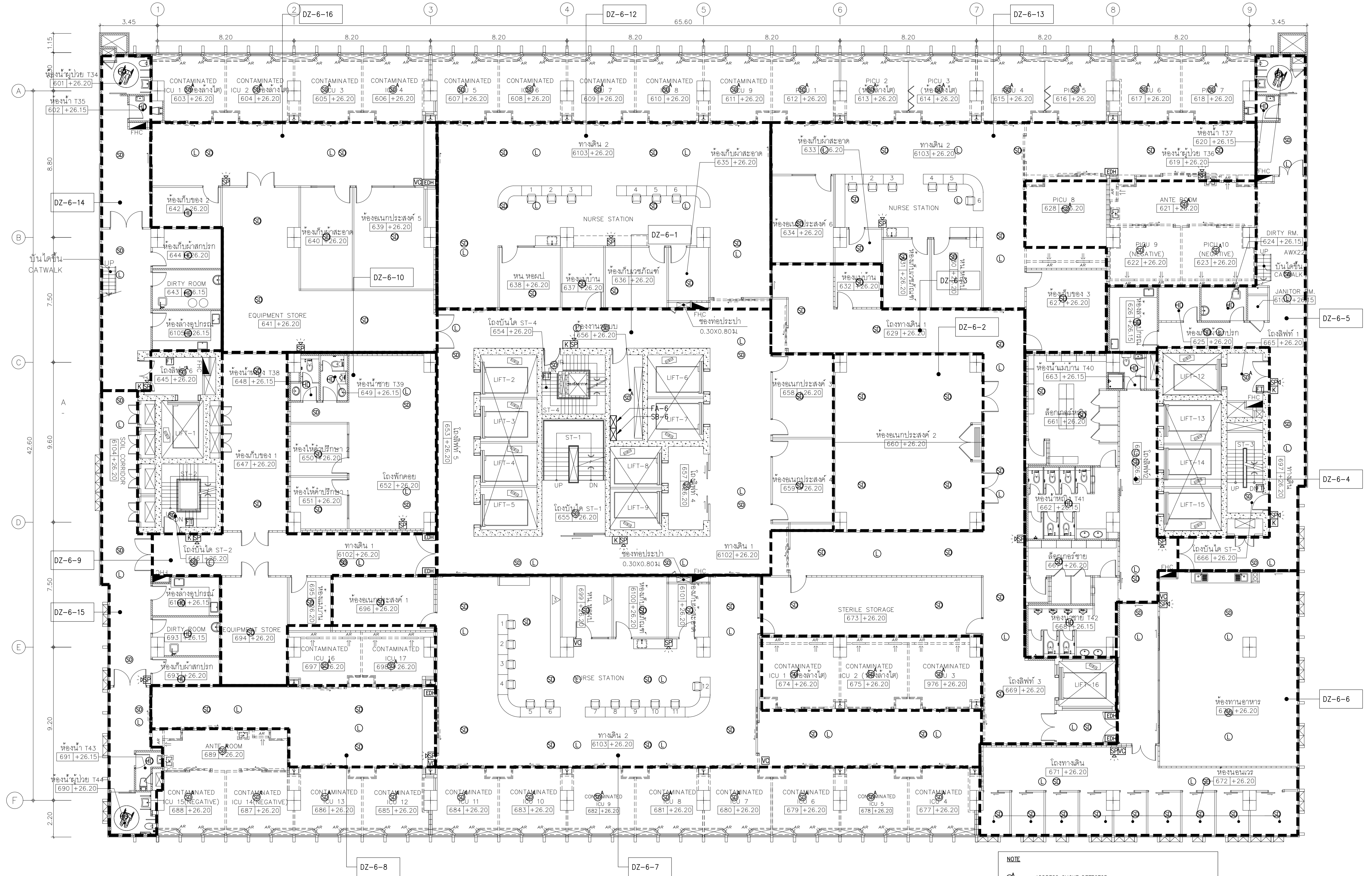
01 แผนระบบแจ้งเหตุเพลิงไหม้และเสียงประกาศชั้นที่ 6 A1@ 1:125 A3@ 1:250 0 2 5 BAR SCALE
