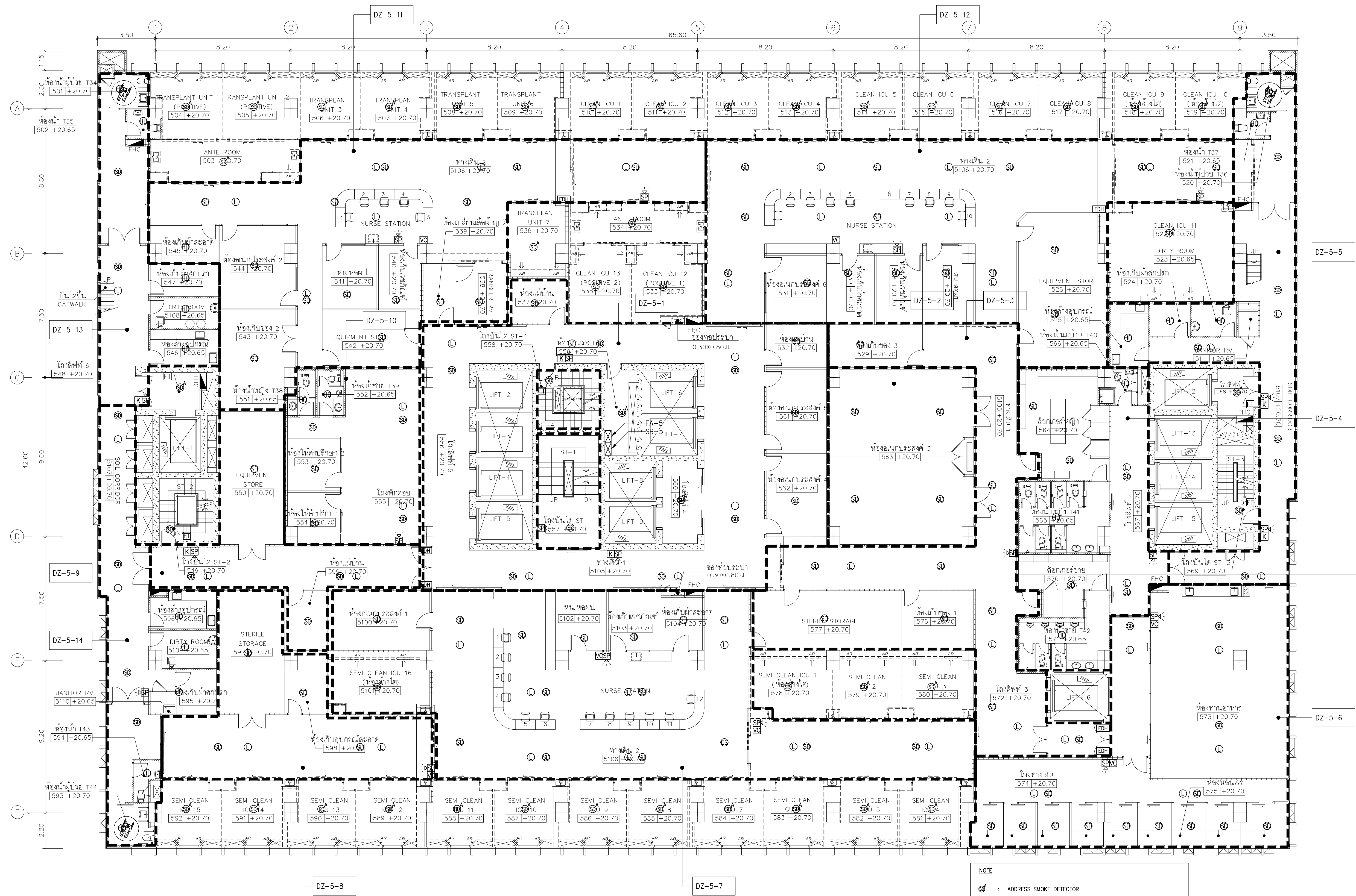
01 แผนระบบแจ้งเหตุเพลิงไหม้และเสียงประกาศชั้นที่ 5
