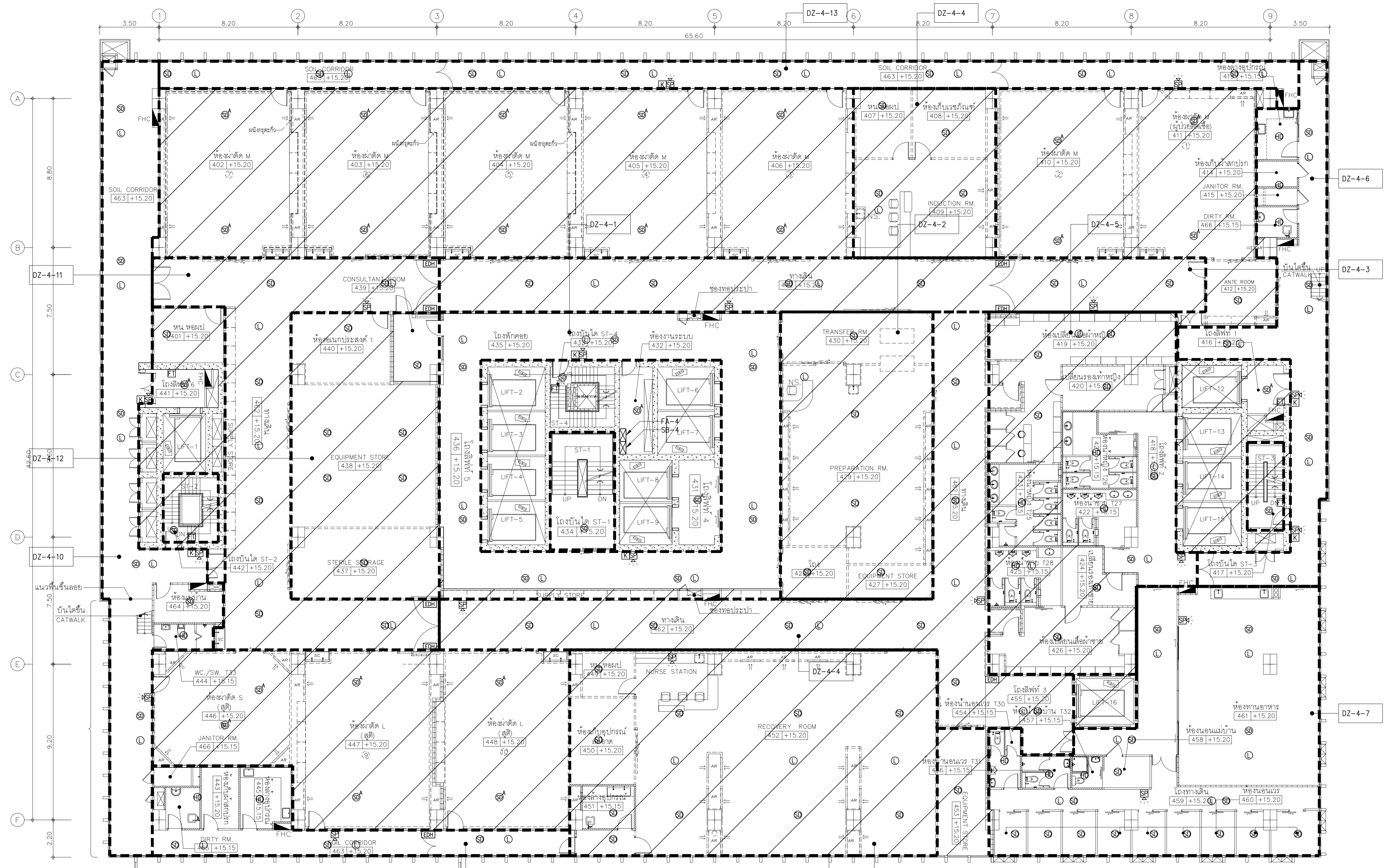
01 แผนระบบแจ้งเหตุเพลิงไหม้และเสียงประกาศชั้นที่ 4 A1@ 1:125 A3@ 1:250
