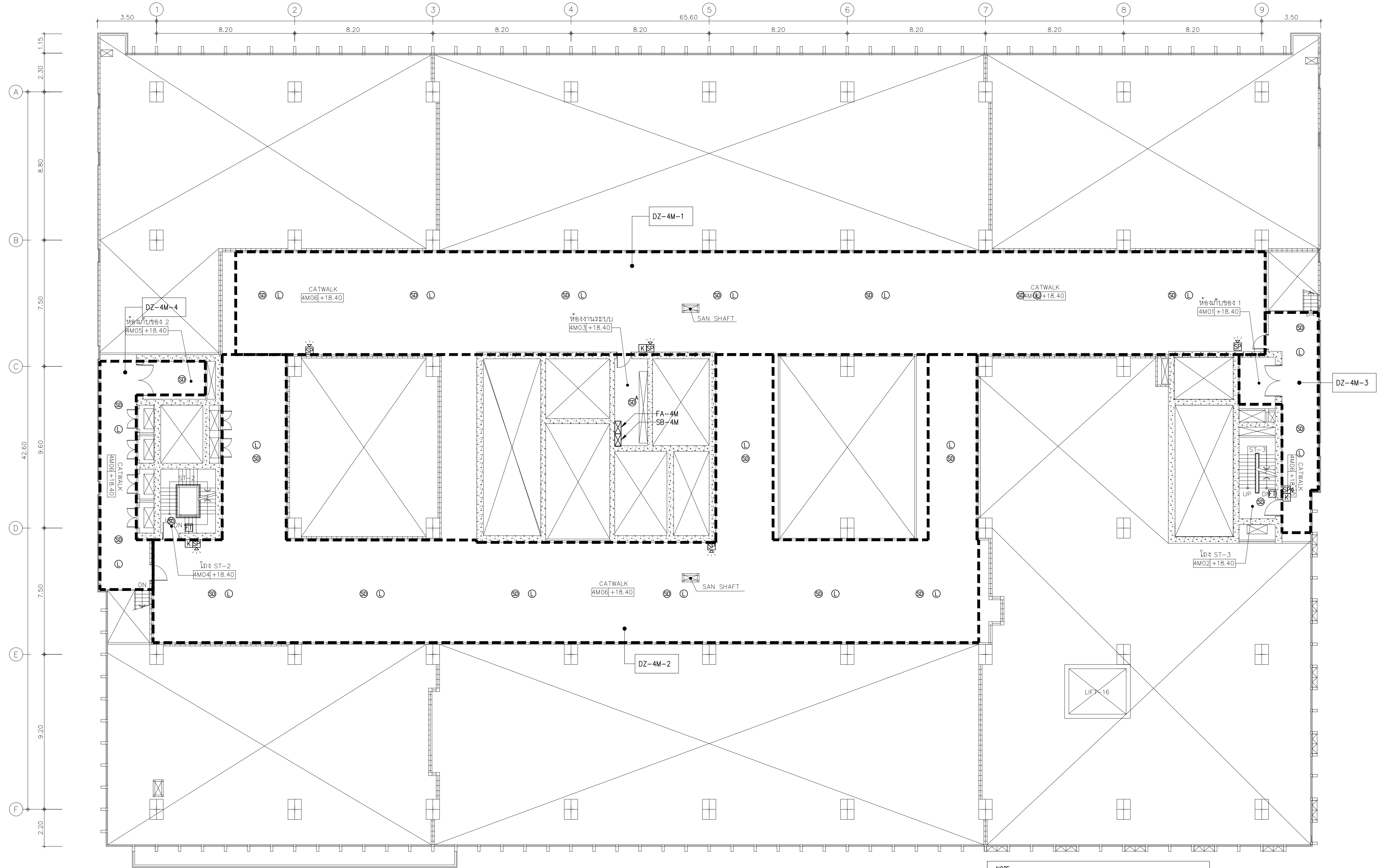
01 แปลนระบบแจ้งเหตุเพลิงไหม้และเสียงประกาศชั้นลอย 4M A1@ 1:125 A3@ 1:250
